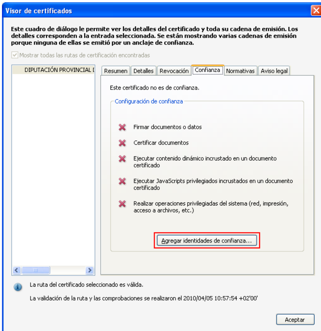
Ilustración 5: Visor de certificados
